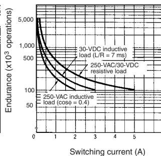
G2R-1Z4, G2R-1AZ4
