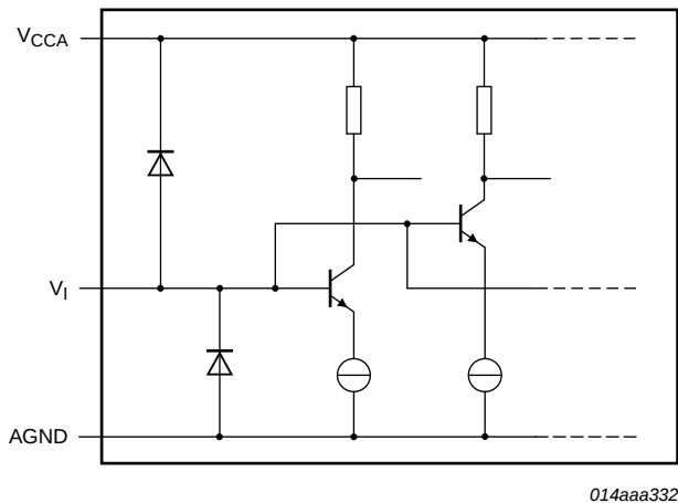
Fig 10. Analog inputs
