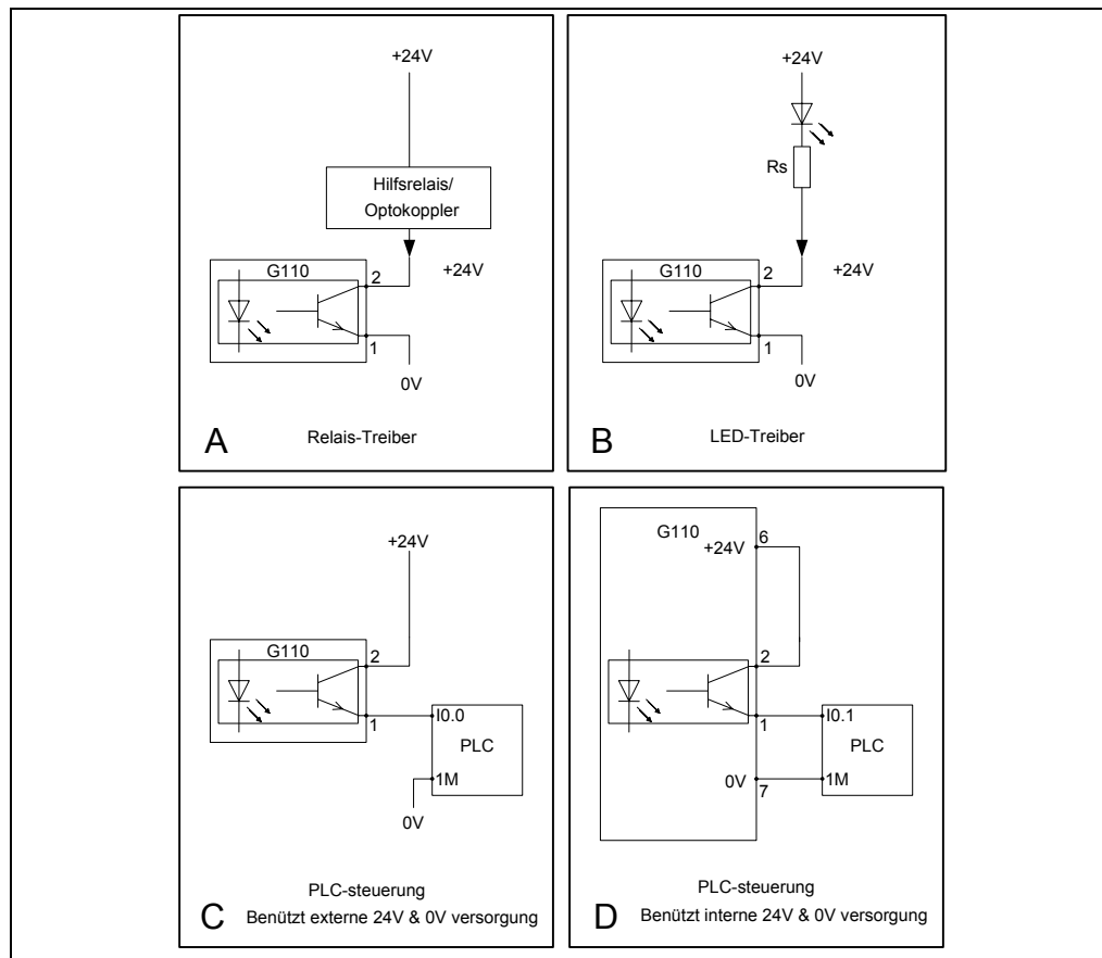
Bild 3-8 Typische Konfigurationen des digitalen Ausgangs
