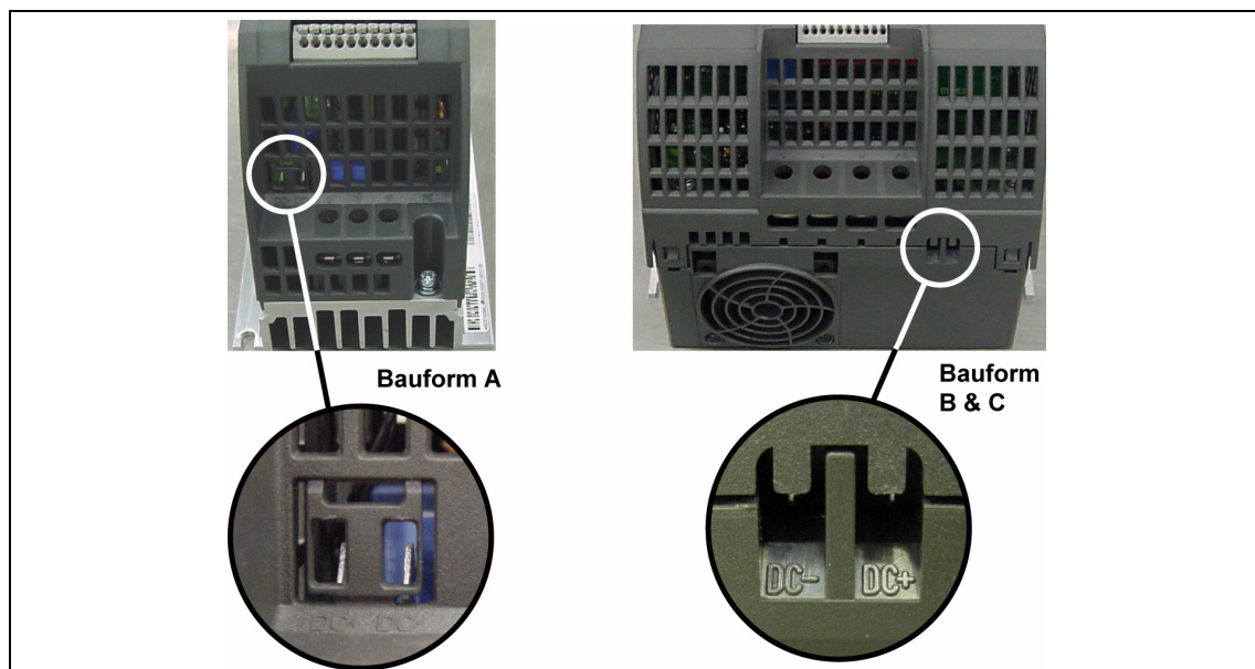
Bild 2-6 SINAMICS G110-DC-Anschlüsse
