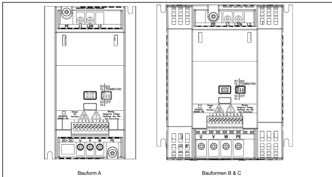
Bild 2-5 SINAMICS G110-Anschlussklemmen
