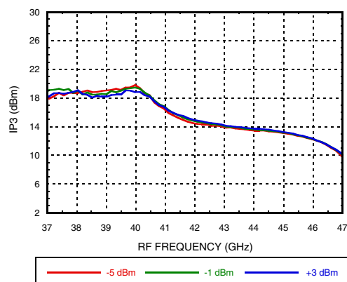
Output IP3 vs. LO Power
