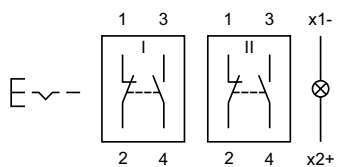
Wiring diagram 24
