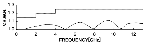
AT-506(40)
