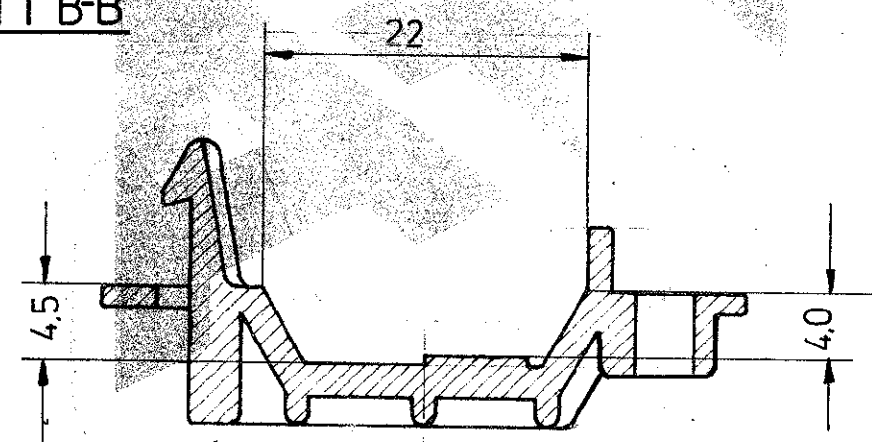
SCHNITT B-B
