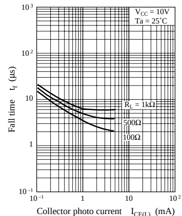
t_f - I_{CE(L)}
