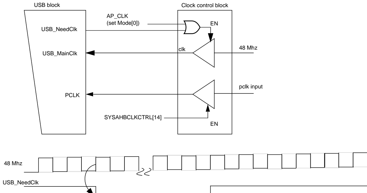
Fig 18. USB clocking
