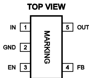
TSOT23-5
