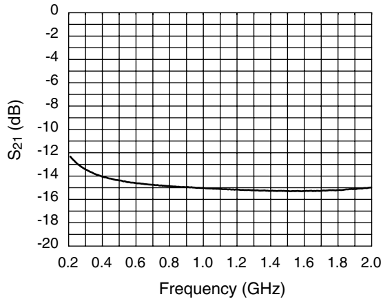
Attenuation
