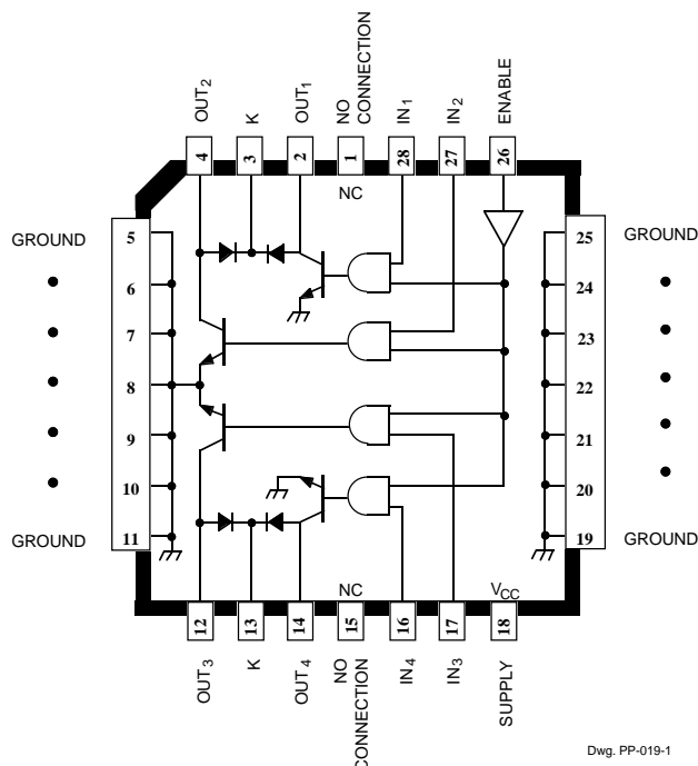
UDN/UDQ2543EB (PLCC)
