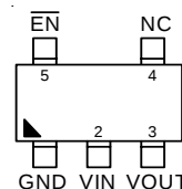
SOT-23-5
