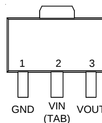
SOT-89
