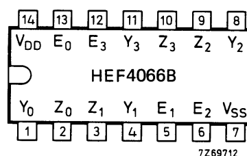
Fig.2 Pinning diagram.
