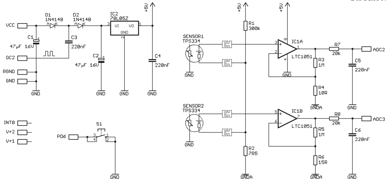
Circuit ARX-SNK
