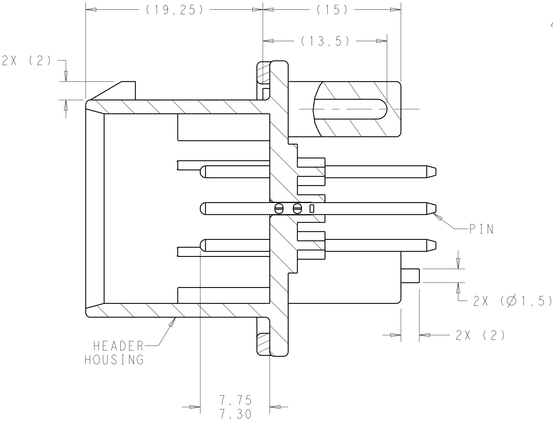
SECTION A-A
