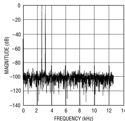
LTC1289 F19
