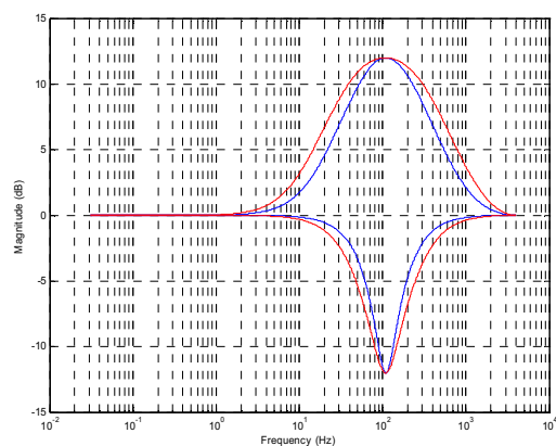
Figure 49 EQ Band 3 – EQ3BW=0, EQ3BW=1
