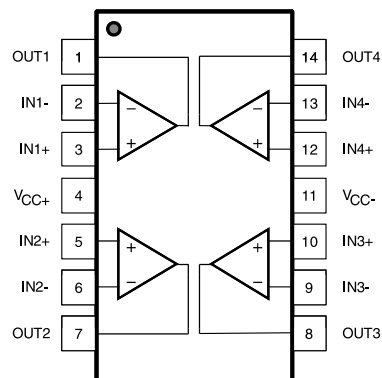
TSSOP14
