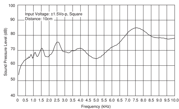
PKMCS0909E4000-R1
