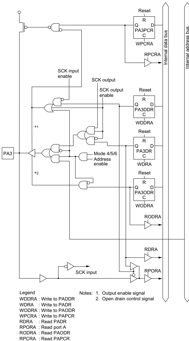
Figure C-5 (d) Port A Block Diagram (Pin PA3)
