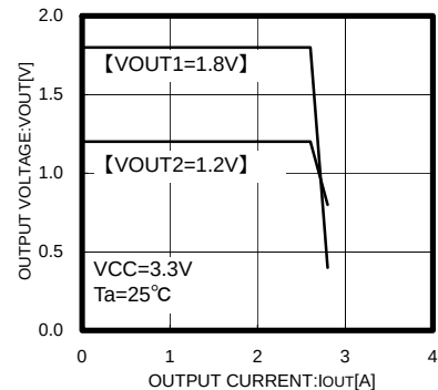
Fig.5 IOUT - VOUT
