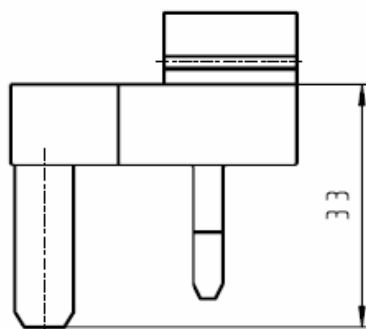
UK-Stecker/plug 1717618
