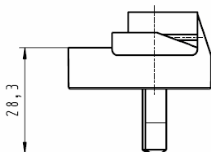
Australien-Stecker/plug 1800496
