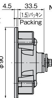
回転角度90° Turning angle
