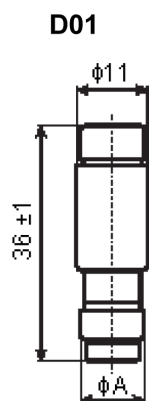
Dimensions : Millimetres
