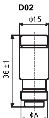
Dimensions : Millimetres
