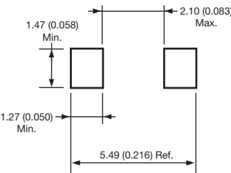
DO-214AC (SMA)
