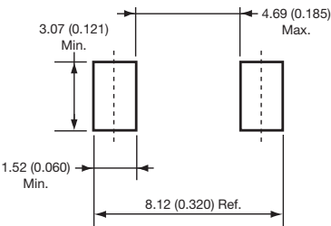
DO-214AB (SMC)
