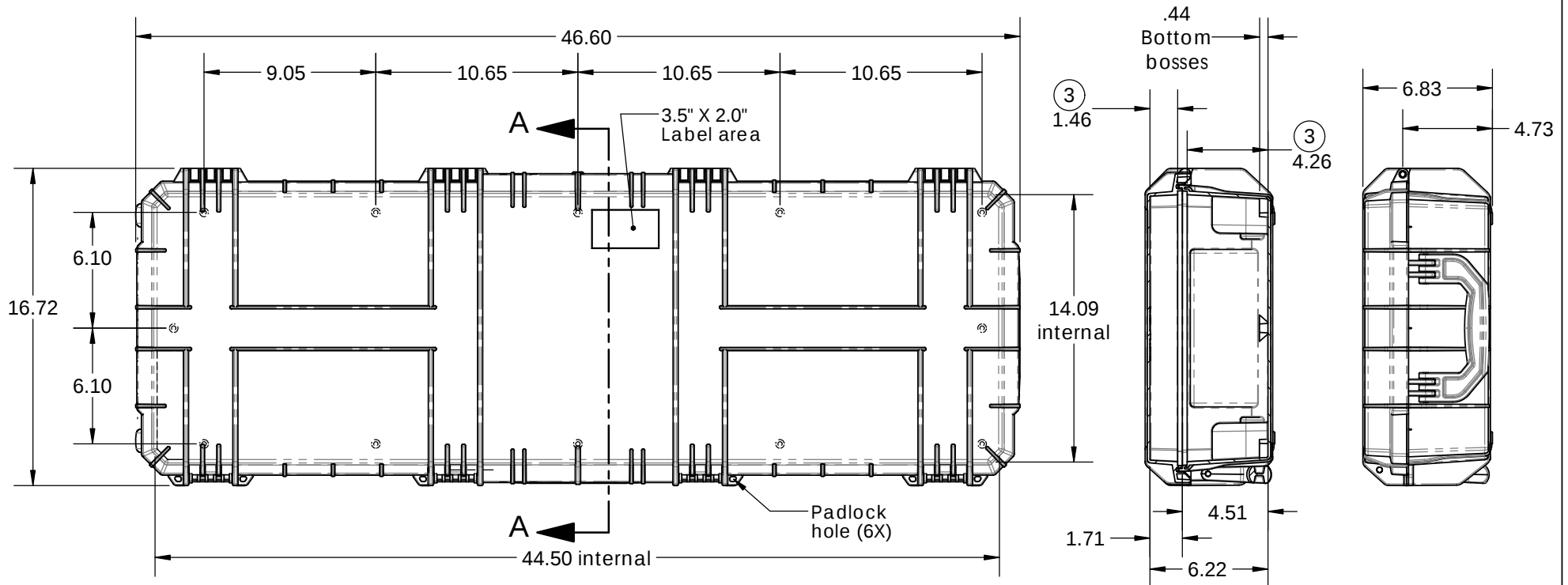
SECTION A-A
