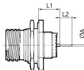
Receptacle type 0
