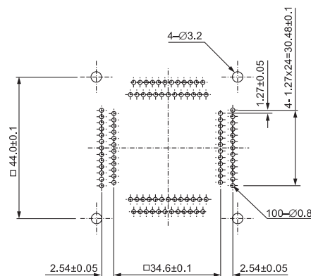
IC51-1004-405-1 (100 Pins)
