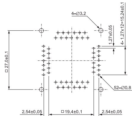
IC51-0524-411-1 (52 Pins)
