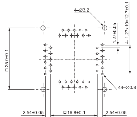
IC51-0444-400 (44 Pins)
