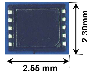
10pinTSON PKG
