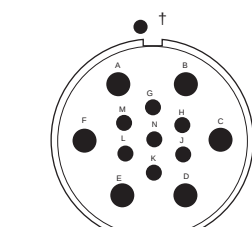
40A33 7 #8(G-N) 6 #4(A-F)
