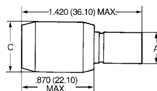
Receptacle
