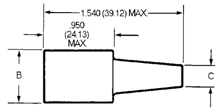
Receptacle P/N 120-1833-000
