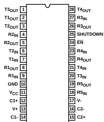
HIN241 (SOIC, SSOP)
