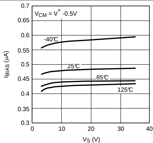
Figure 27. I_{\text{BIAS}} vs. V_{\text{S}}
