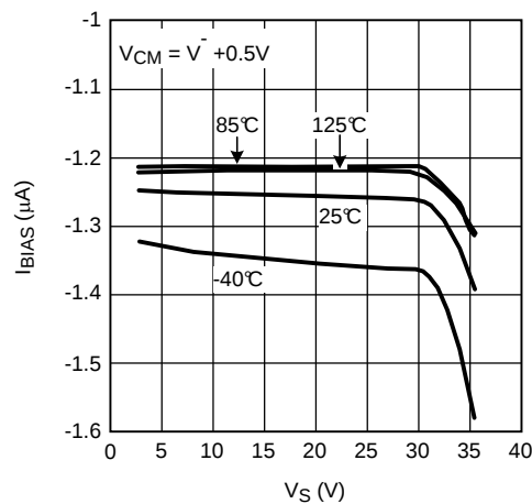
Figure 26. I_{\text{BIAS}} vs. V_{\text{S}}
