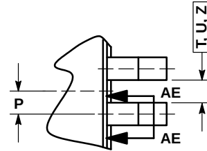
DETAIL Y
