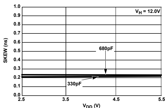
FIGURE 31. tSkewF vs V DD
