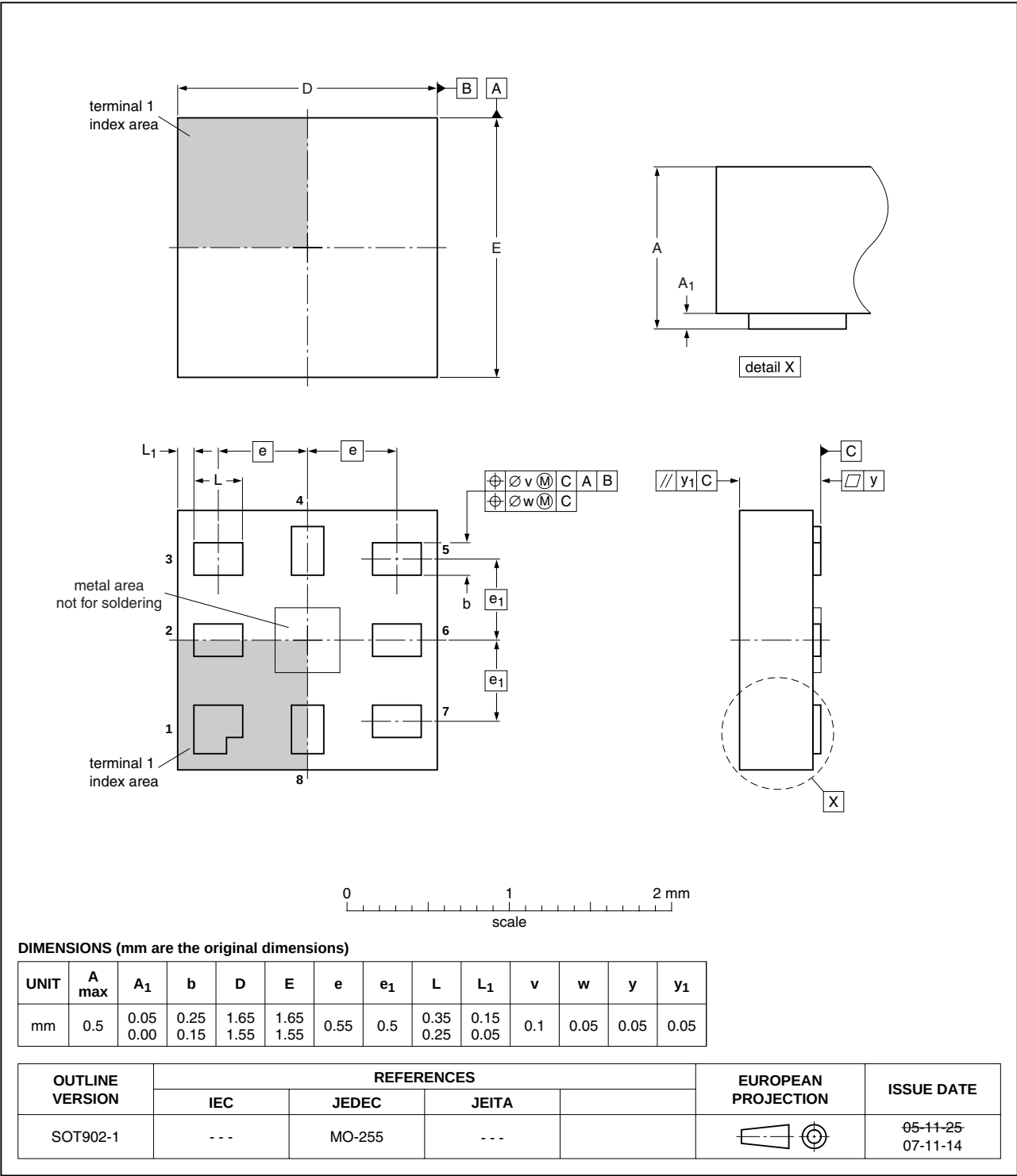
Fig 21. Package outline SOT902-1 (XQFN8U)
