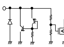
23pin&lt;EN &gt;
