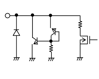
15pin&lt;OC&gt;
