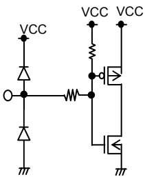
7pin&lt;PERST_IN#&gt;
