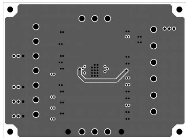
Mid Layer 2
