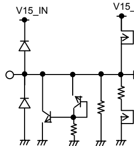
8,9pin&lt;V15_1,V15_2&gt;
