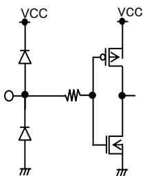
12pin&lt;CPUSB#&gt;
