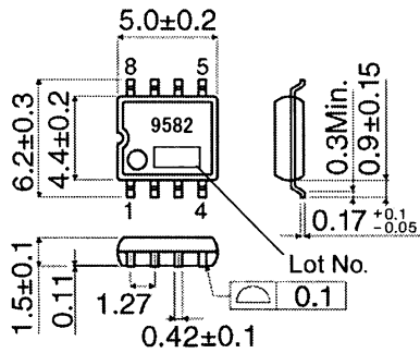
Fig.1 SOP8
