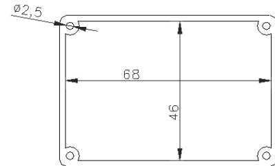
Gehäuseoberteil
