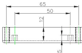
Gehäuseunterteil
