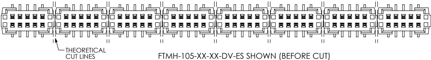
FTMH-105-XX-XX-DV-ES SHOWN (BEFORE CUT)
