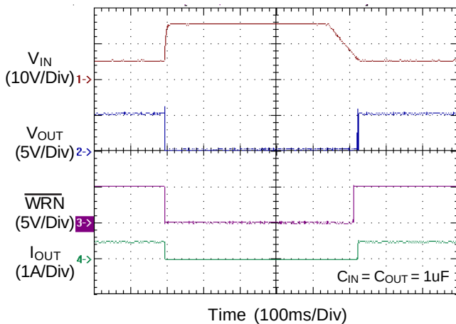
Input OVP
