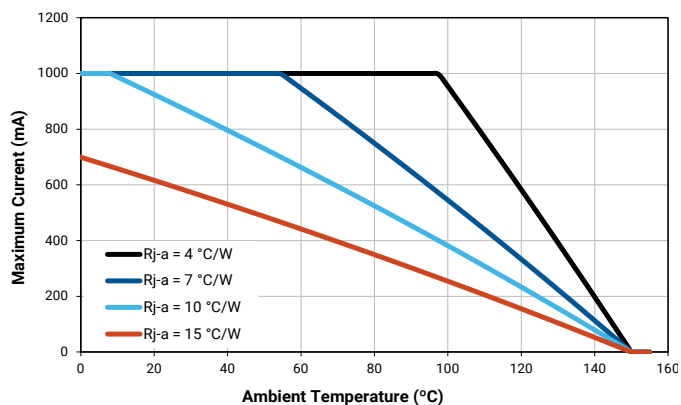
XLamp XM-L EZW LED, 12-V
