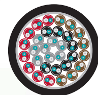
Schnittzeichnung
