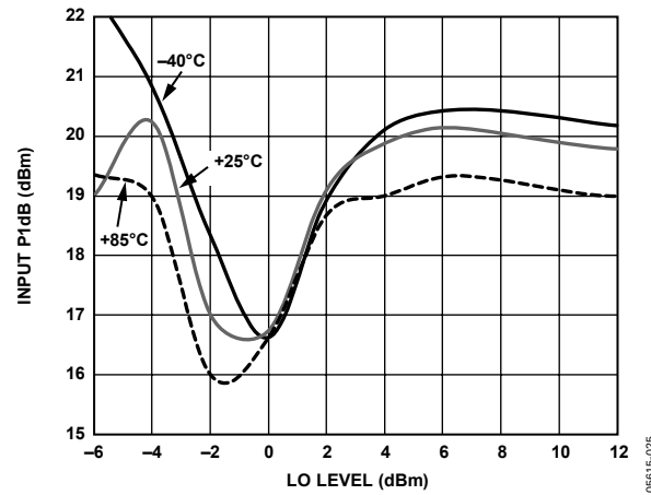
Figure 25. Input P1dB vs. LO Level
