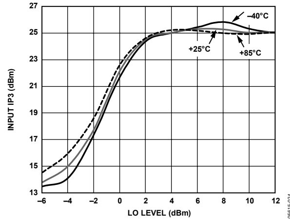
Figure 24. Input IP3 vs. LO Level
