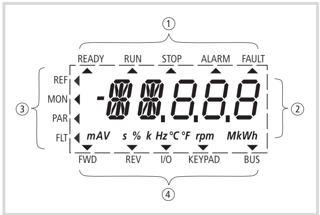
Abbildung 64: LCD-Anzeige (Bereiche)
