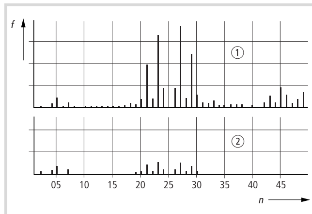
Abbildung 134: Hochfrequente Anteile der Ausgangsspannung
