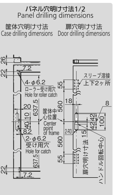
A-462-1-1R (右開き用) Right-hand use
