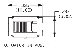
ACTUATOR IN POS. 1
