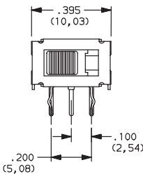
ACTUATOR IN POS. 1
