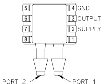
MS4525-DSvxxxxP
