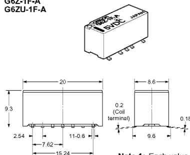
G6Z-1F-A G6ZU-1F-A
